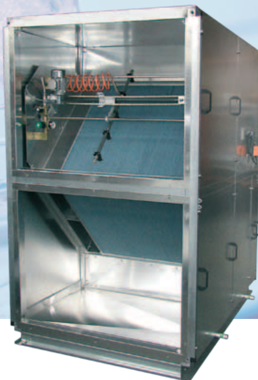
3D lekbak met condensafvoer
