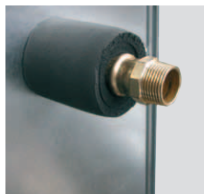
Doorvoering met Armaflex-isolatie
