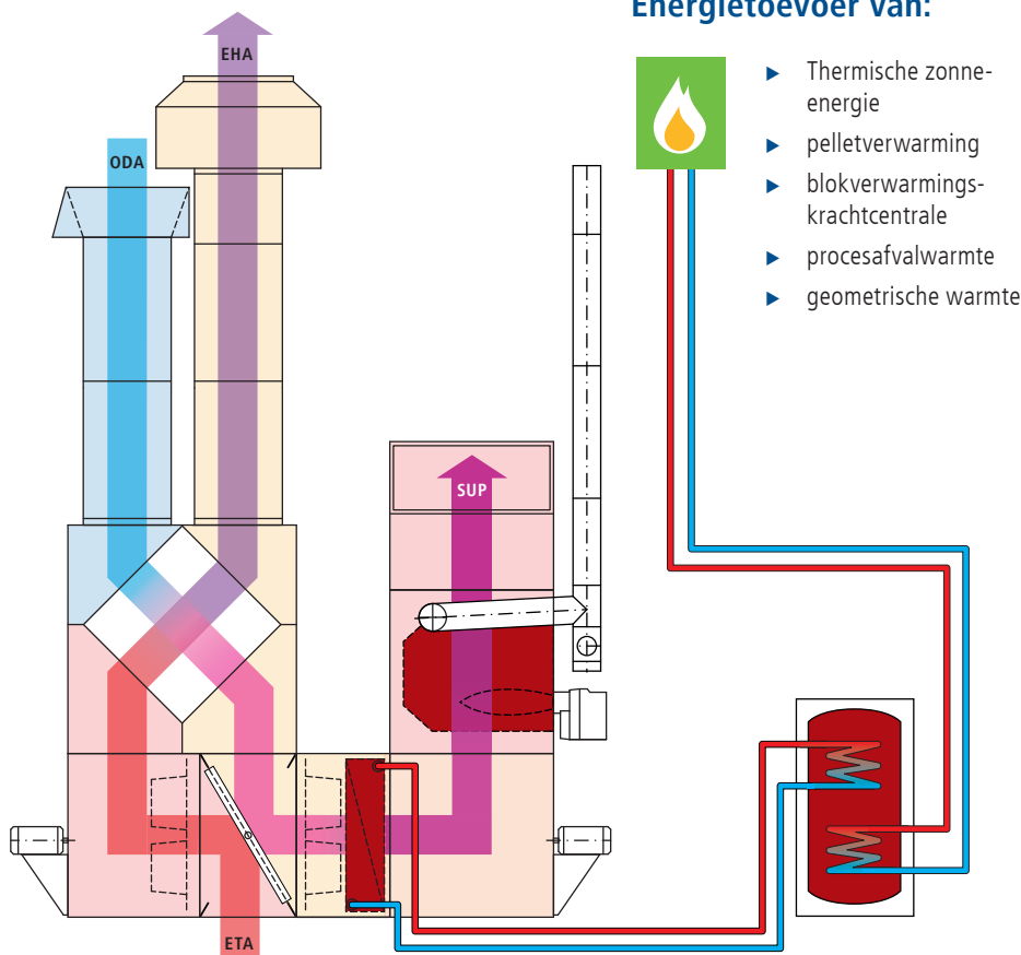
Spuitinstallatie-aggregaat met extra register voor het gebruik van regeneratieve energie
